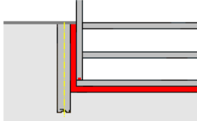
Grundwasserabdichtung Waterproofing below groundwater table
